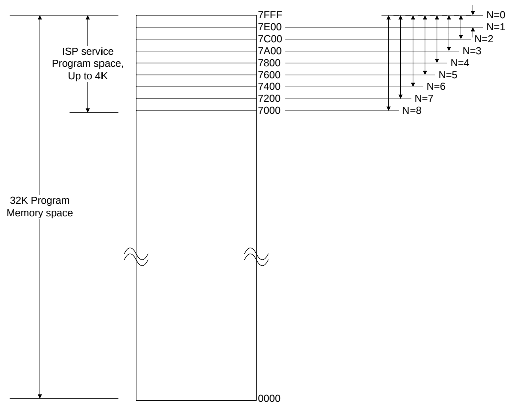
图 3-1: SM5958 programmable Flash
